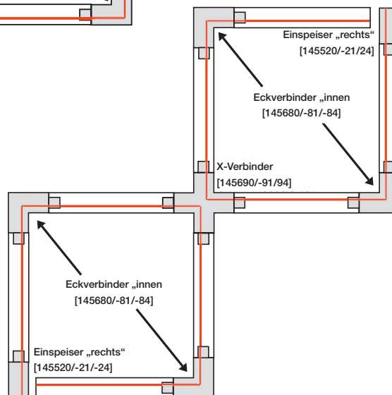
Beispiel 3 [2 Stromkreise]
